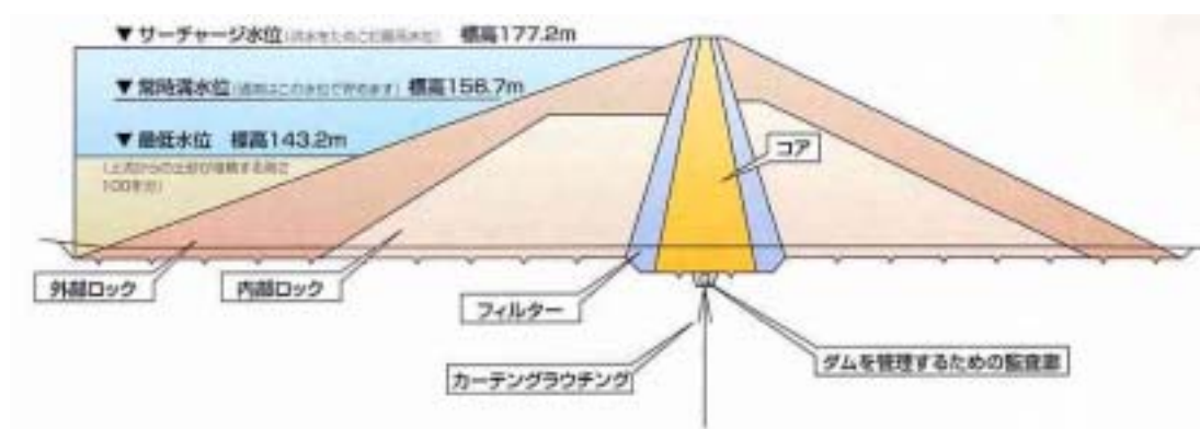
図 6 - 7 森吉山ダム標準断面図
