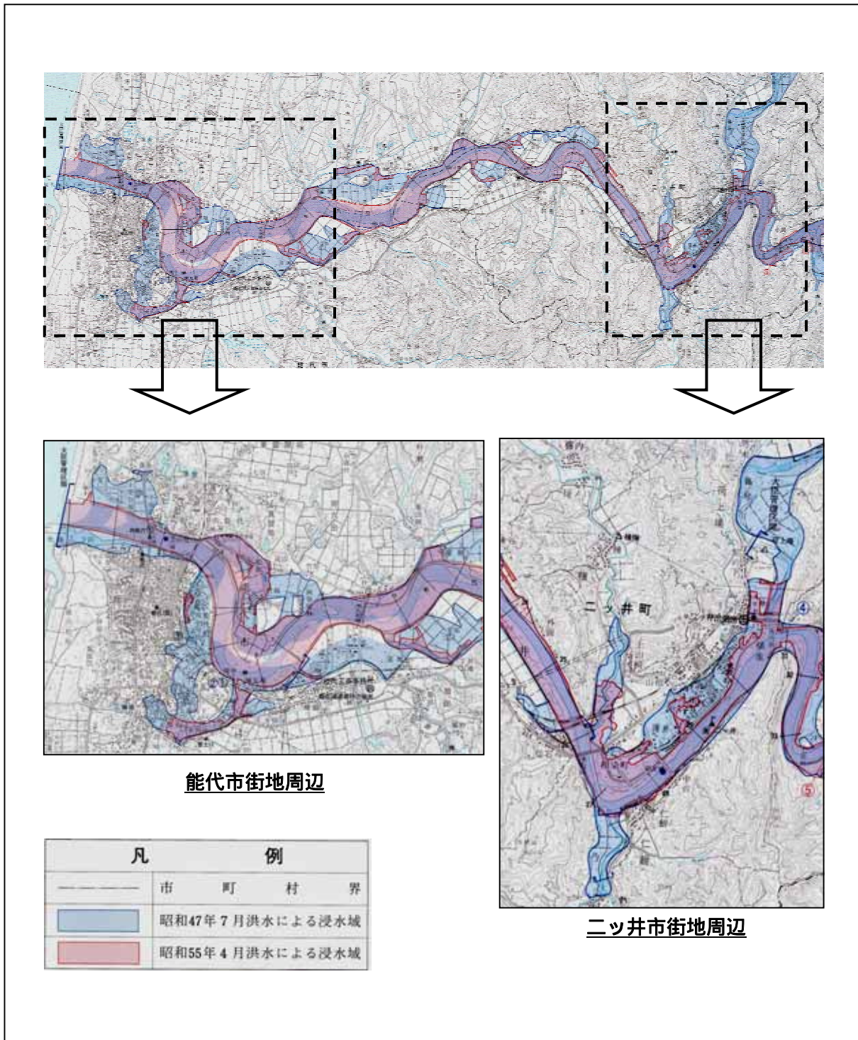
図 2 - 8 S47.7月,S55.4月洪水浸水実績図
