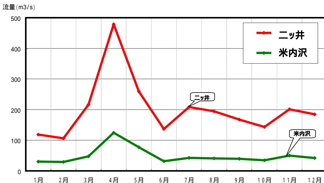
図2-5 主要観測所 月別平均流量 (S45~H15)
