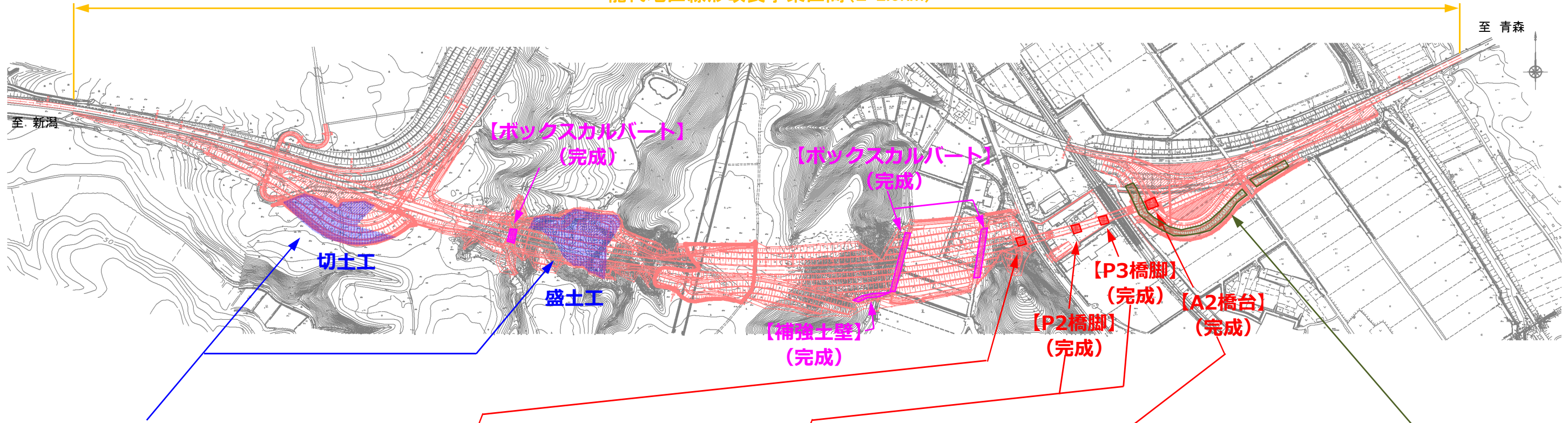
【本線切土盛土区間】 写真はR2.12.15撮影
