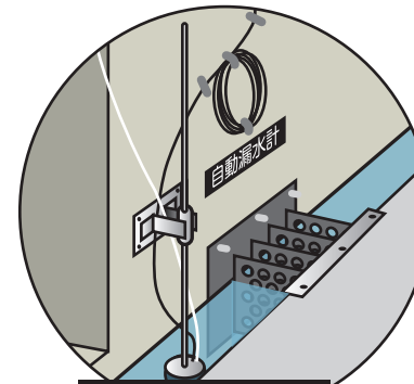
漏水計
