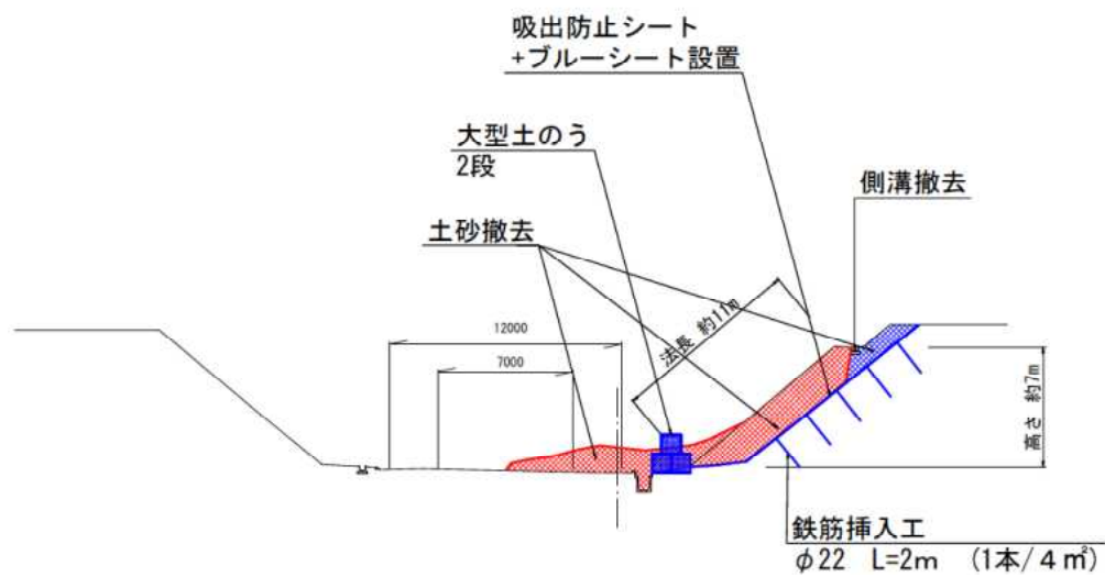
横断図
