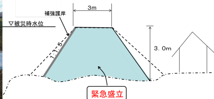
堤防復旧断面
