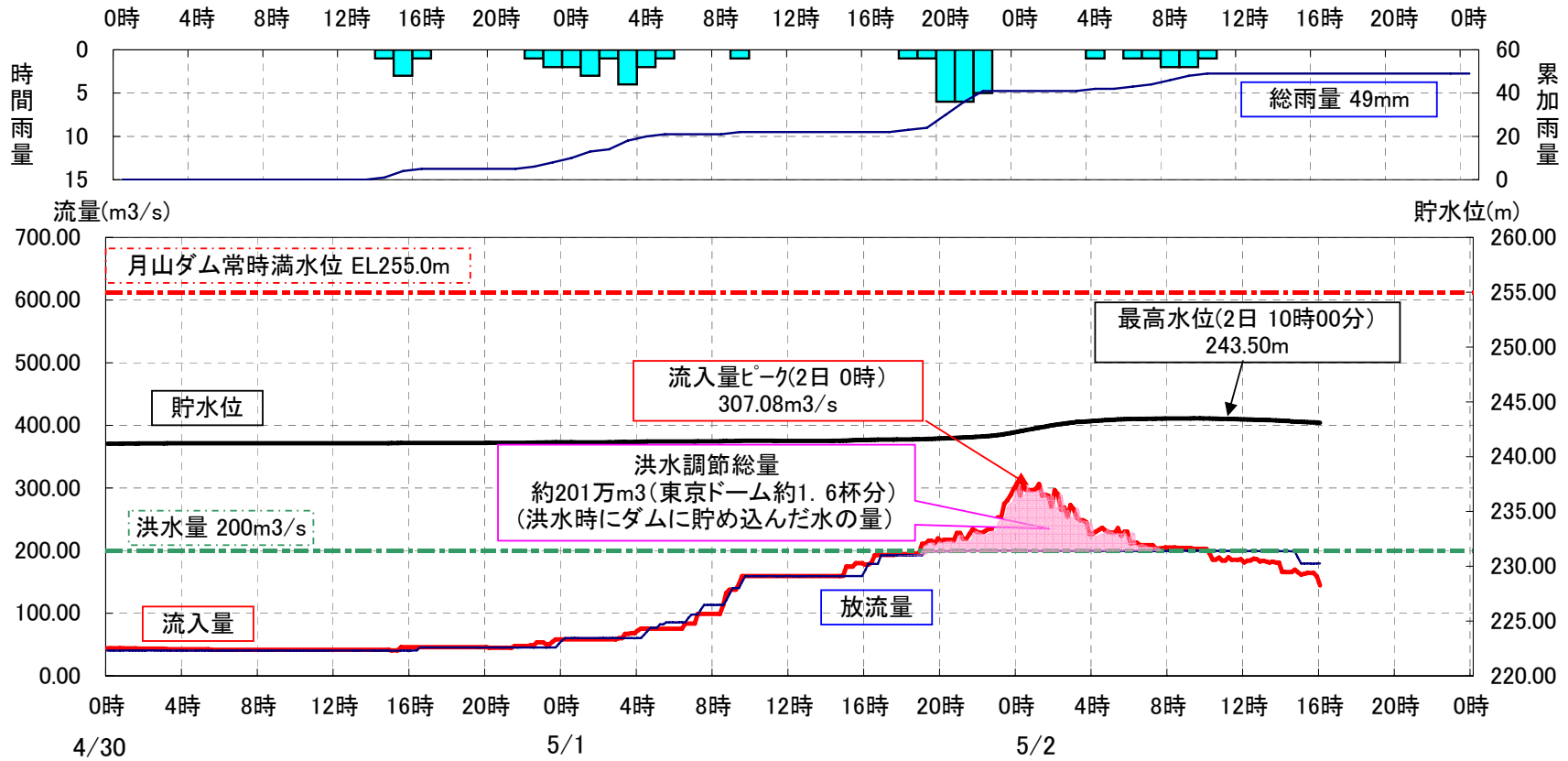
月山ダム洪水波形(h23.5.1)
