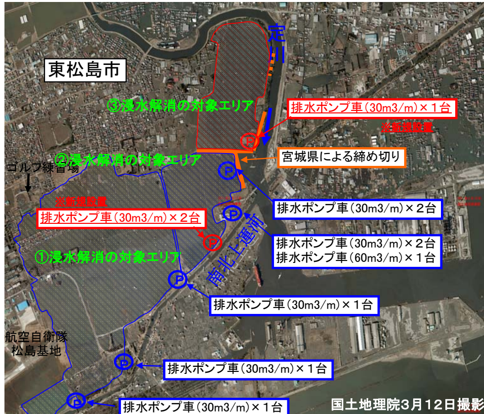
東松島市大曲地区、浸水解消エリア 現在、排水ポンプ車合計 11台で排水中。 (排水能力:1時間で25mプール約54個分、約21,600m 3 )
