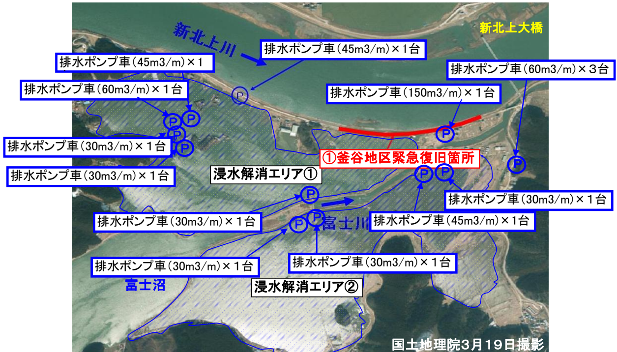
石巻市釜谷地区 浸水解消エリア 現在、排水ポンプ車合計 14台で排水中。 (排水能力:1時間で25mプール約107個分、約42,300m 3 )
