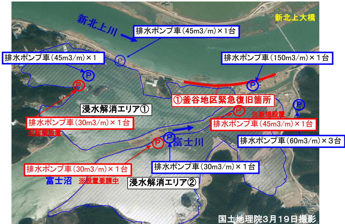
石巻市釜谷地区 浸水解消エリア 4月5日排水ポンプ車増強 3台
