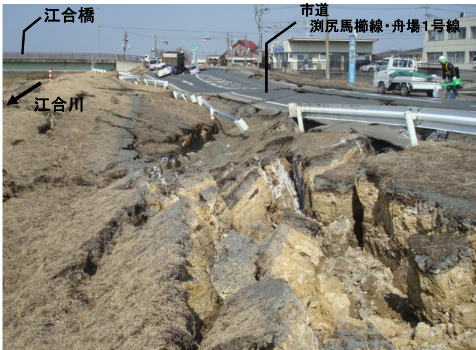
3月11日 堤防被害状況 堤防亀裂・沈下
