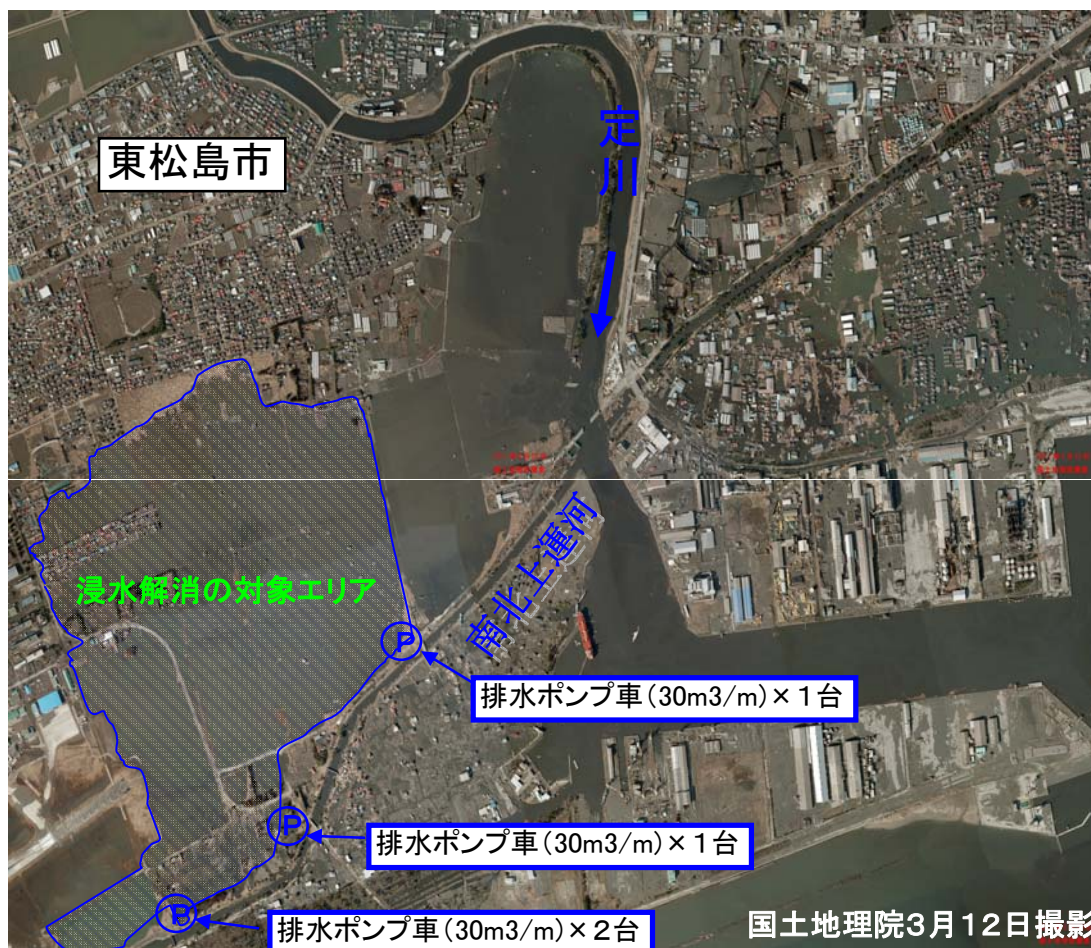
浸水解消のため、東松島市大曲付近に排水ポンプ車を設置し排水作業を実施。(東松島市大曲地先)
