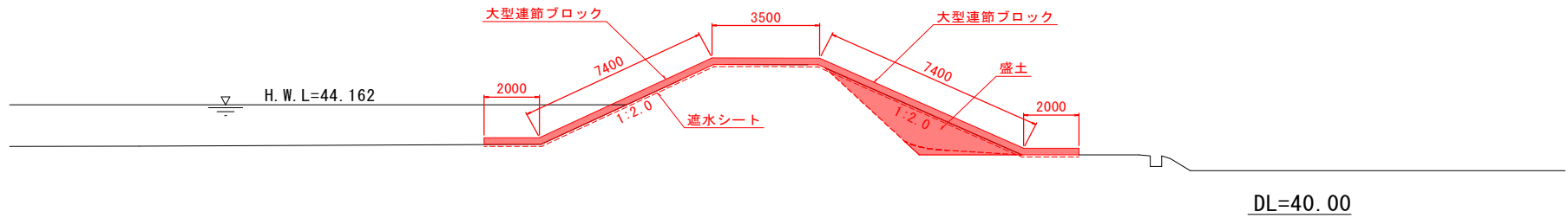
横断図 鯉川6.4k
