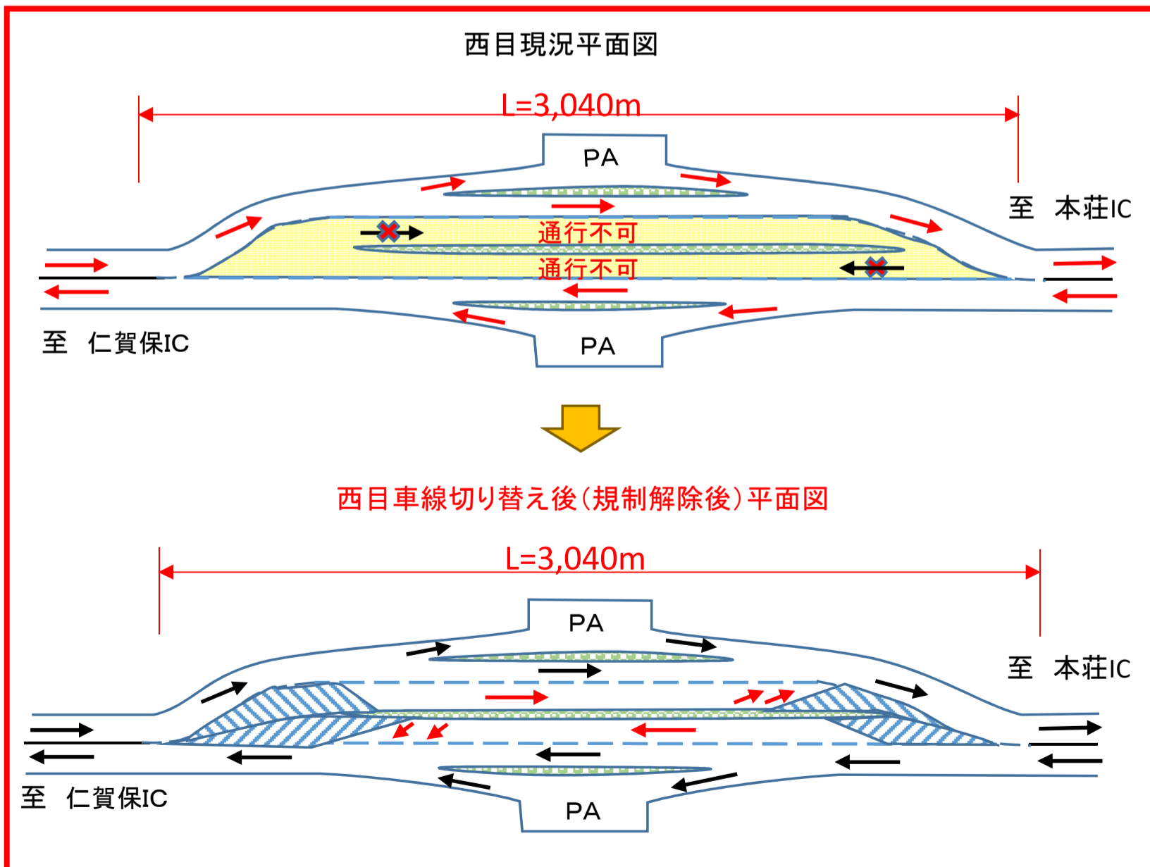
◎車線切り替え後平面図
