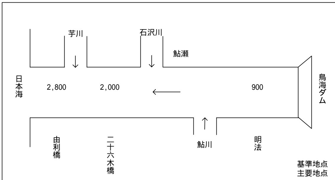
図 4-1 子吉川における河道の目標流量
