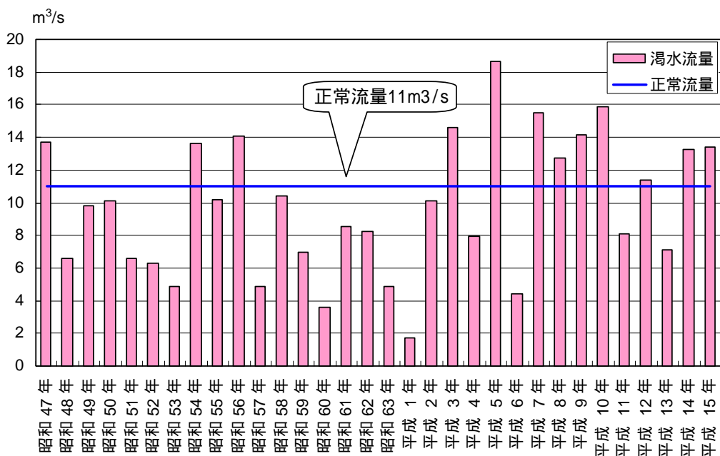
図 3-7 各年渇水流量と正常流量 (宮内地点)
