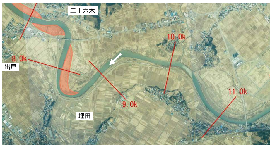
図 5-9 河道掘削位置図 (7.0～11.0k)
