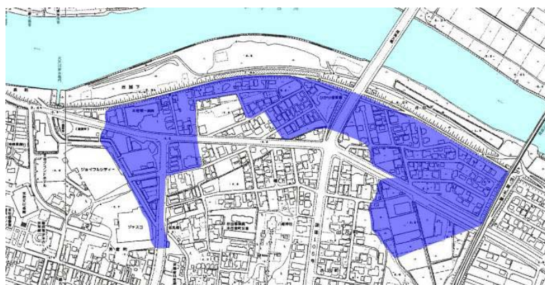
図 5-13 大沢川排水機場による排水効果(平成14年4月洪水)
